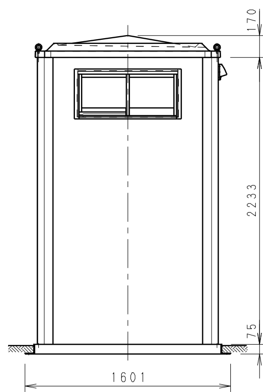
右側面
