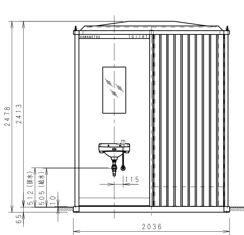
正面図
