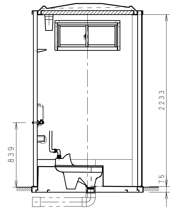
B-B' 断面図
