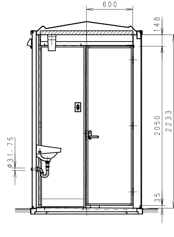
A-A' 断面図
