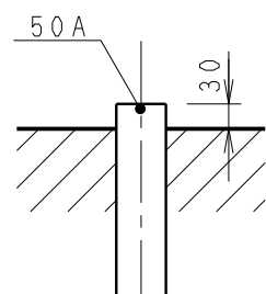
50A (小便排水) 基礎面より30
