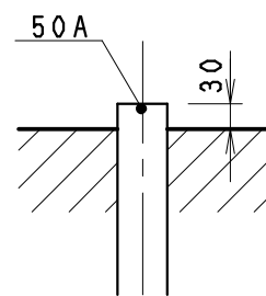
50A (小便排水) 基礎面より30
